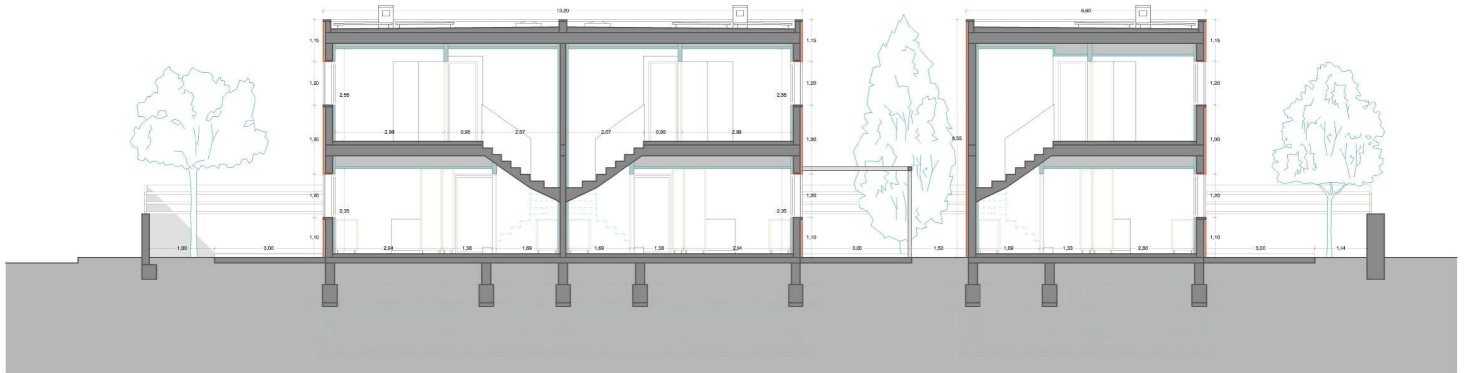
Sección 2
