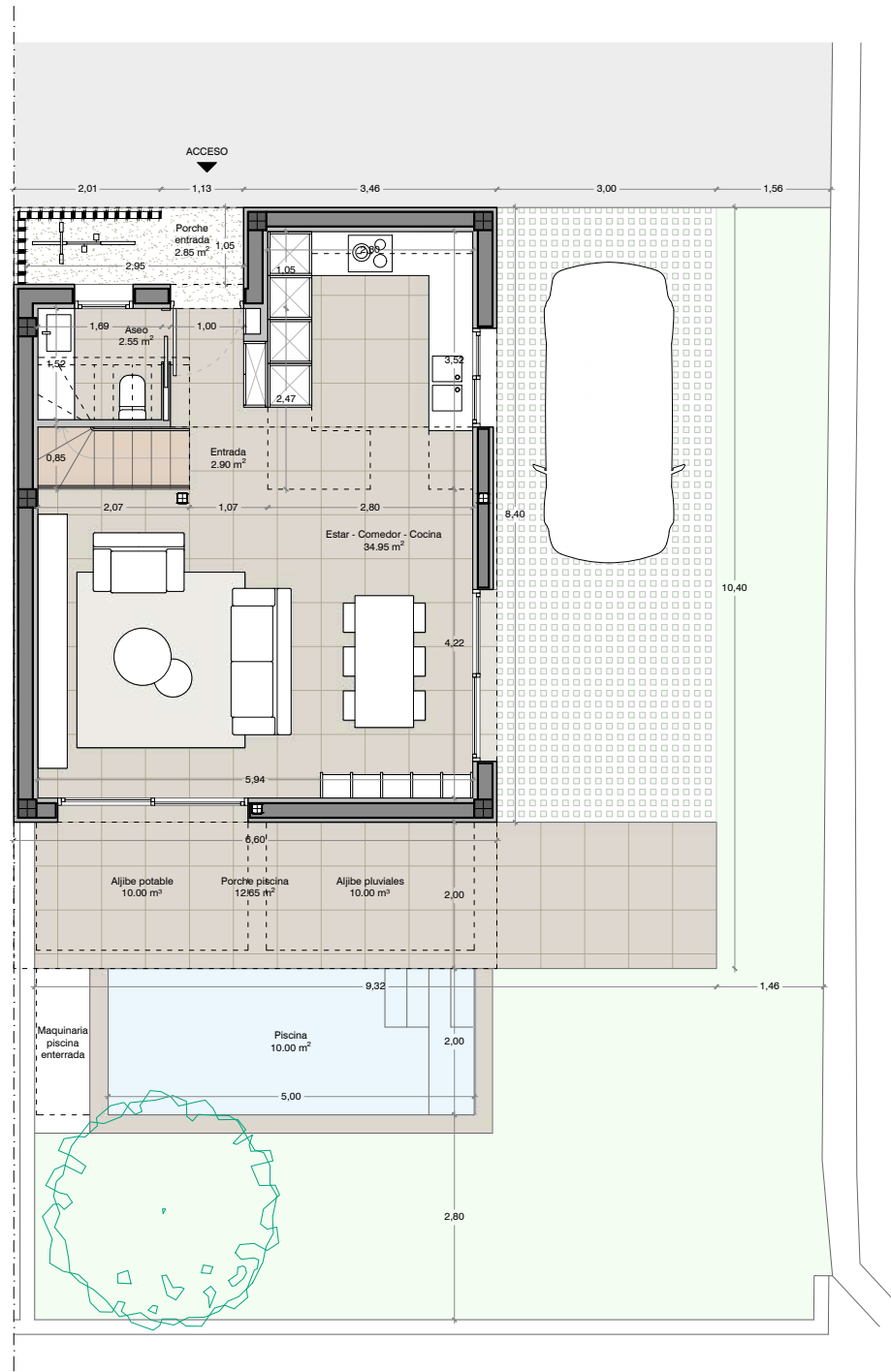
Planta baja
