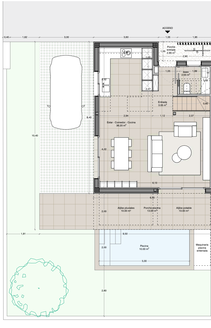
Planta baja
