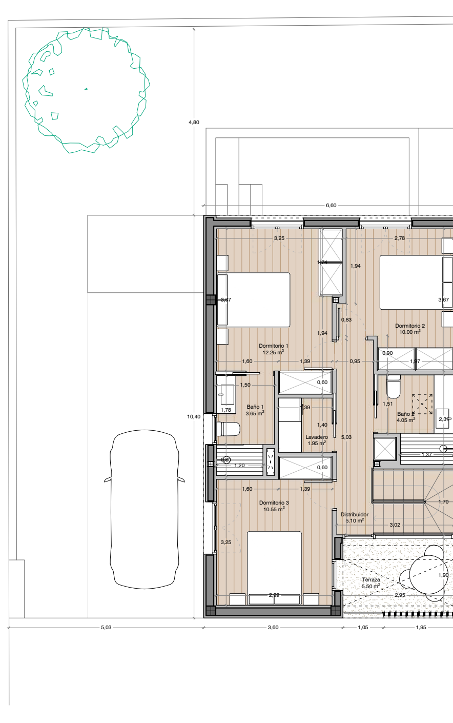
Planta piso
