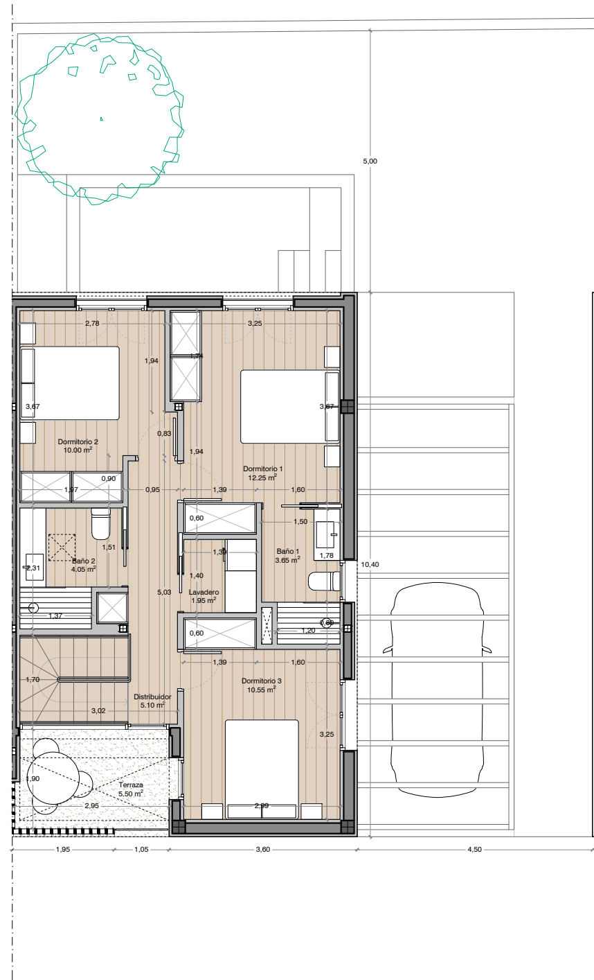
Planta piso
