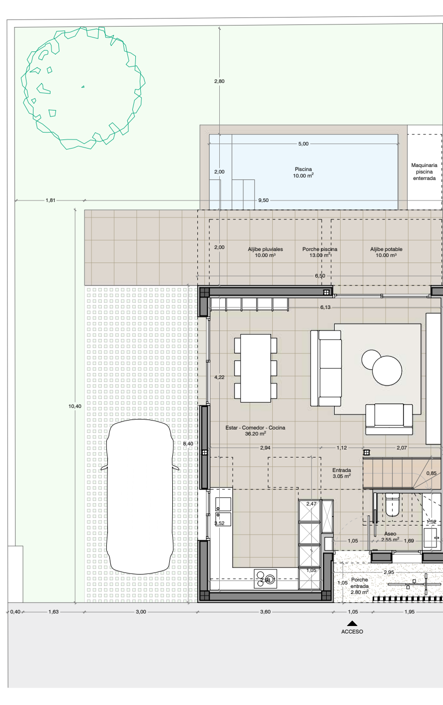
Planta baja
