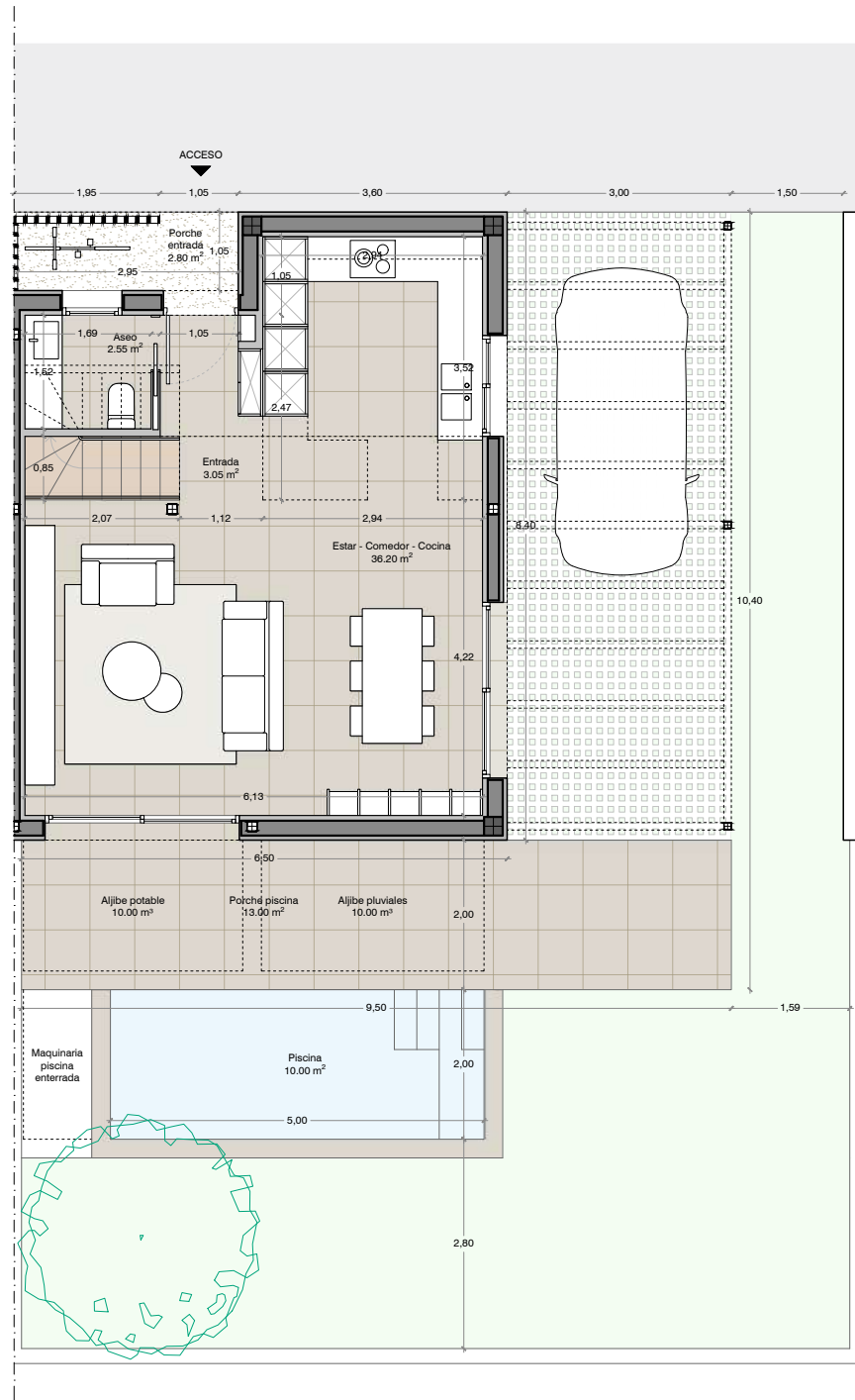
Planta baja
