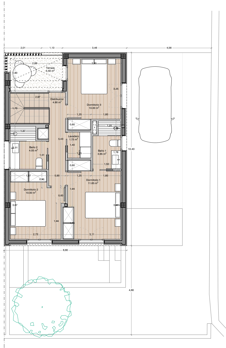
Planta piso
