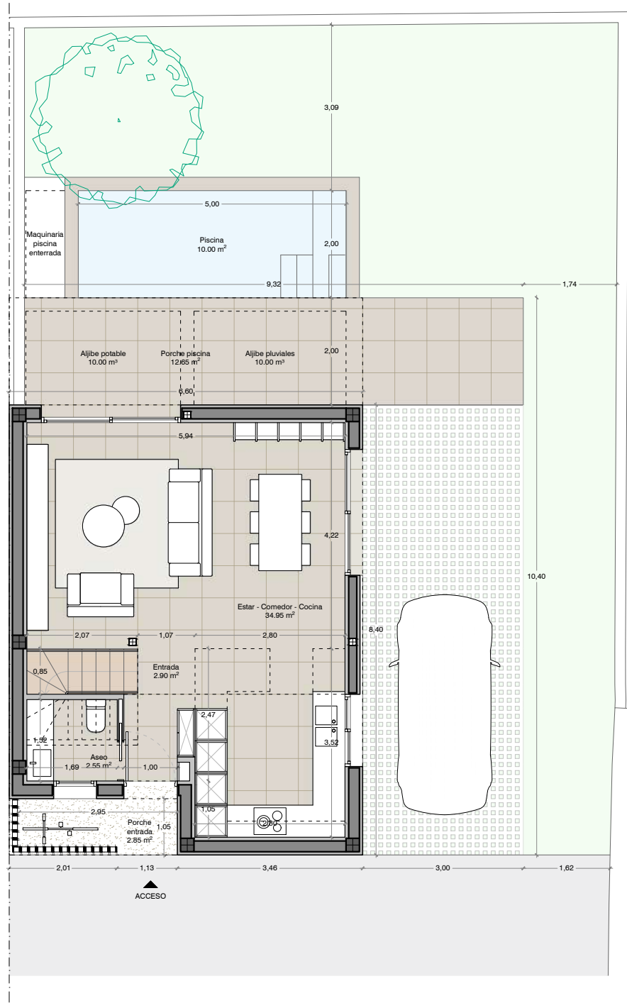
Planta baja
