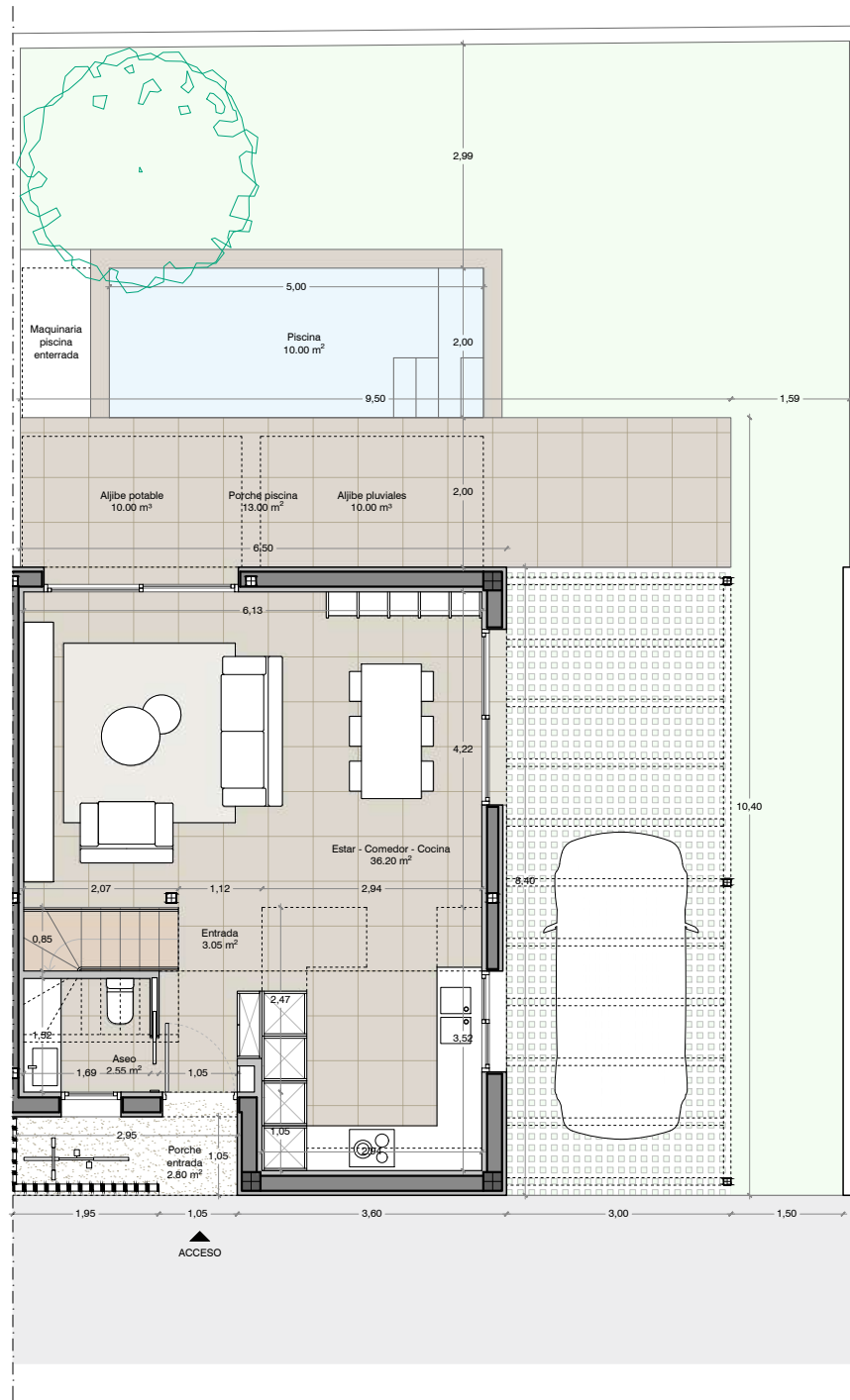
Planta baja
