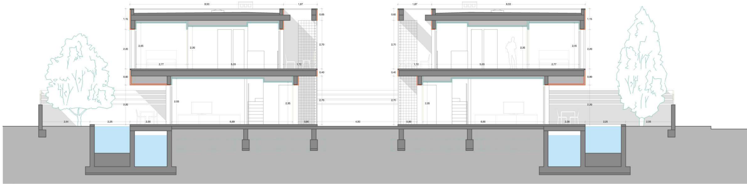
Sección 1
