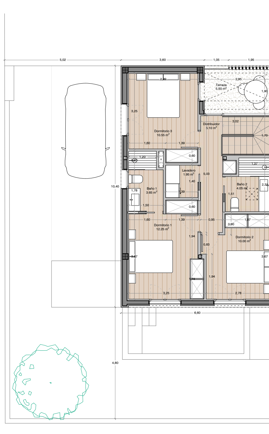
Planta piso
